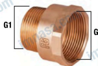
G1: EN 10226 / 1 (BS21) G: ISO 228/1 (BS2779)
